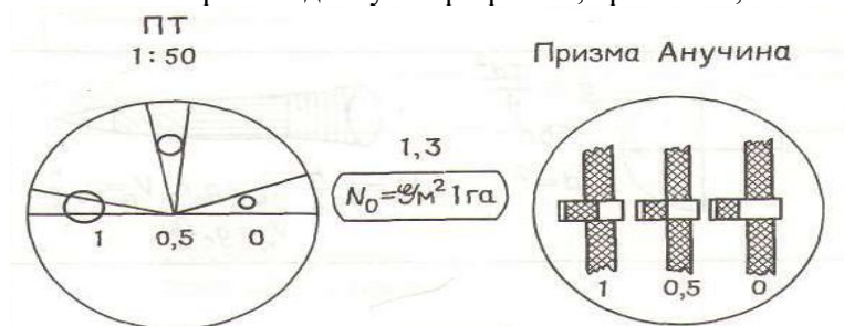
Рис. 4 Таксационный прицел (призма) Н.П. Анучина
