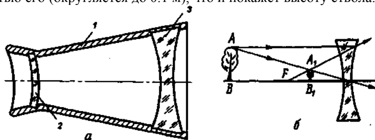
Рис.2 - Оптический высотомер Н.П.Анучина
