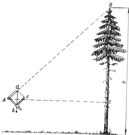
Рис. 1 Измерение высоты дерева мерной вилкой
